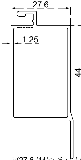
دفعه منخل مع كنت (27.6 / 44) ملم الرقم التسلسلي للصنف: BLT3569 الوزن 0.597:(Kg/m)
