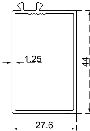
سادة لتحتون 27.5 ملم الرقم التسلسلي للصنف: BLT3510 الوزن 0.507:(Kg/m)
