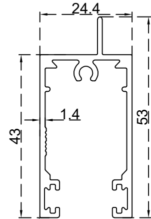
تحتون دفة مع فرشائيتين 24.4 ملم الرقم التسلسلي للصنف: BLT3316 الوزن 0.628:(Kg/m)
