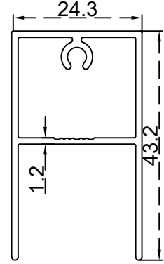
عليون دفة 24.6 ملم الرقم التسلسلي للصنف: BLT841 الوزن 0.464:(Kg/m)
