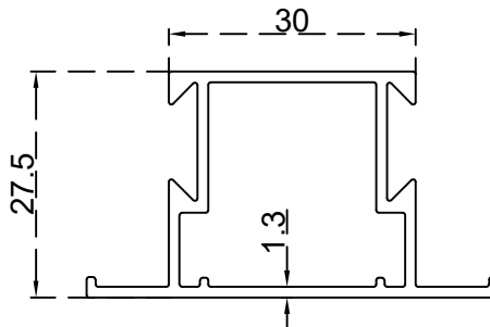
قاطع دفة زجاج الرقم التسلسلي للصف: BLT465 الوزن 0.555:(Kg/m)
