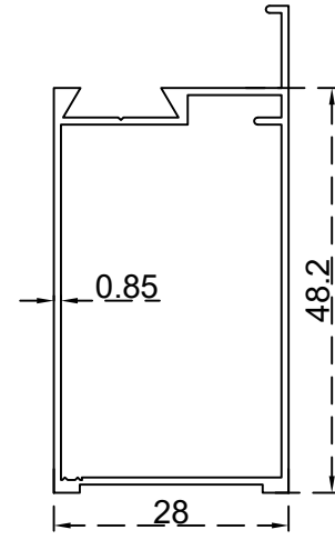
دفة زجاج (28 / 48.2) ملم الرقم التسلسلي للصف: BLT052 الوزن 0.430:(Kg/m)
