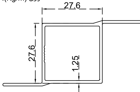
سيما الرقم التسلسلي للصنف: BLT494 الوزن 0.302:(Kg/m)
