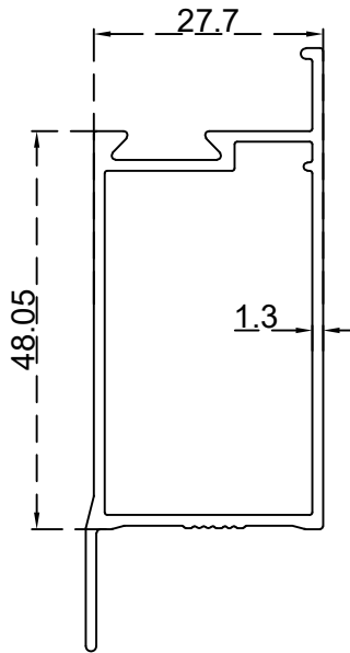
دفة زجاج مع كنت (27.7 / 48.05) ملم الرقم التسلسلي للصف: BLT3721 الوزن 0.667:(Kg/m)
