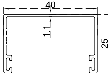
جنب مجرى واحد الرقم التسلسلي للصف: BLT3570 الوزن 0.309:(Kg/m)
