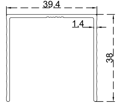
عليون مجرى واحد 38 ملم الرقم التسلسلي للصنف: BLT3624 الوزن 0.406:(Kg/m)
