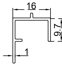
بي عادي الرقم التسلسلي للصنف: BLT1808 الوزن 0.131 : (Kg/m)
