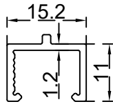
بي كيس الرقم التسلسلي للصنف: BLT3306 الوزن 0.135 : (Kg/m)
