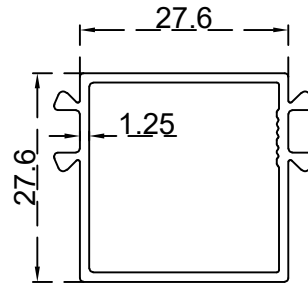
قاطع طولي لتحتون 27.5 ملم الرقم التسلسلي للصنف: BLT3314 الوزن 0.423 : (Kg/m)
