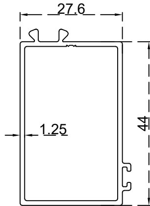
شوليف بي كبس لتحتون 24.6 ملم الرقم التسلسلي للصنف: BLT3509 الوزن 0.520:(Kg/m)
