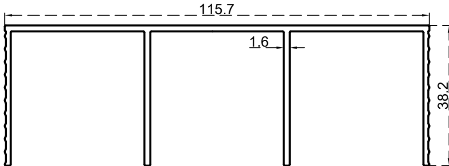
عليون ثلاث مجاري 38 ملم الرقم التسلسلي للصنف: BLT839 الوزن 1.092:(Kg/m)
