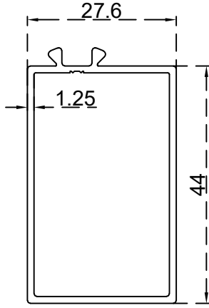
سادة لتحتون 24.6 ملم الرقم التسلسلي للصنف: BLT3312 الوزن 0.501:(Kg/m)
