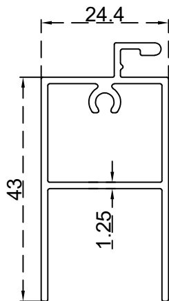
تحتون عليون منخل 24.4 ملم الرقم التسلسلي للصنف: BLT3151 الوزن 0.546 : (Kg/m)
