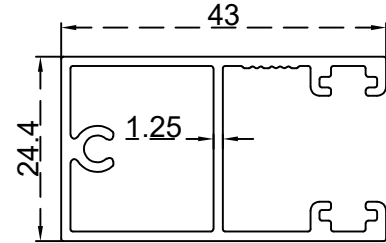
عليون دفة مع فرشائيتين 24.4 ملم الرقم التسلسلي للصنف: BLT3307 الوزن 0.580:(Kg/m)
