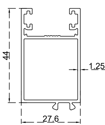
سادة لتحتون 27.5 ملم الرقم التسلسلي للصنف: BLT3311 الوزن 0.599:(Kg/m)
