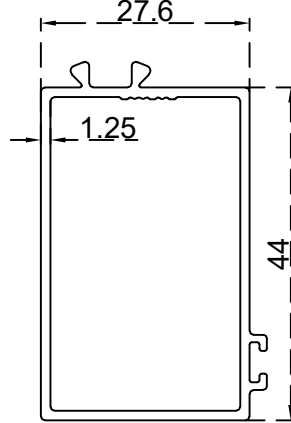
شوليف بي كبس لتحتون 27.5 ملم الرقم التسلسلي للصنف: BLT3797 الوزن 0.526:(Kg/m)
