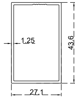
سادة (1.25*43.6*27.1)ملم الرقم التسلسلي للصنف: BLT3323 الوزن 0.460:(Kg/m)
