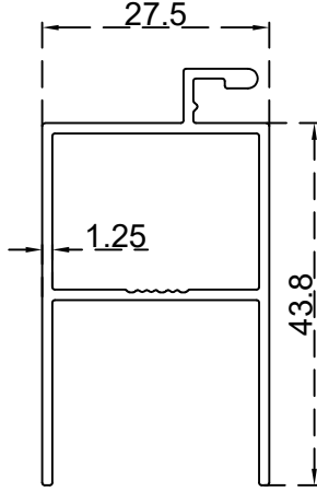
تحتون عليون منخل 27.5 ملم الرقم التسلسلي للصنف: BLT3630 الوزن 0.523:(Kg/m)
