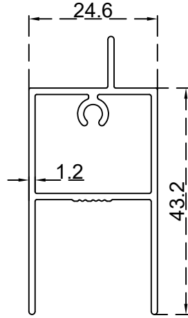
تحتون دفة 24.6 ملم الرقم التسلسلي للصنف: BLT842 الوزن 0.506:(Kg/m)
