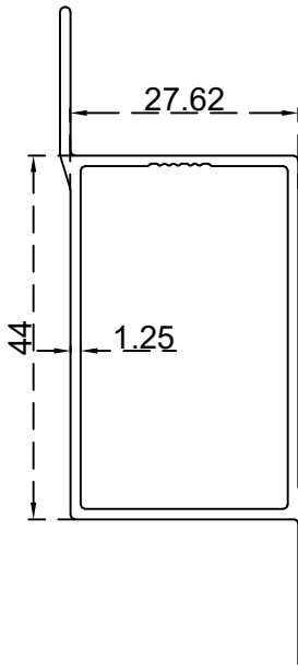
دفة (27.6 / 44) ملم مع كنتين الرقم التسلسلي للصف: BLT3489 الوزن 0.602:(Kg/m)
