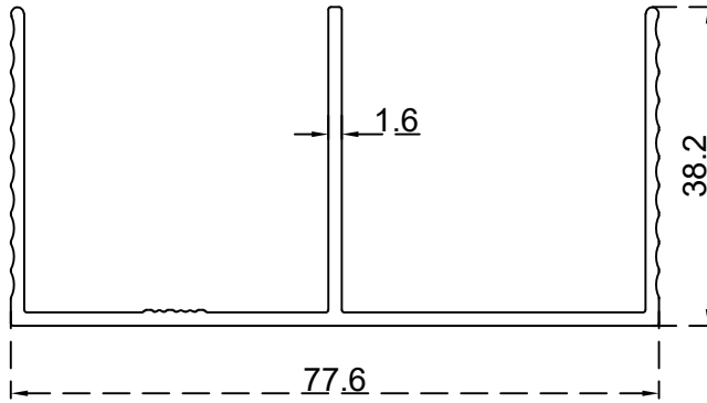
عليون مجريين 38 ملم الرقم التسلسلي للصنف: BLT840 الوزن 0.770:(Kg/m)
