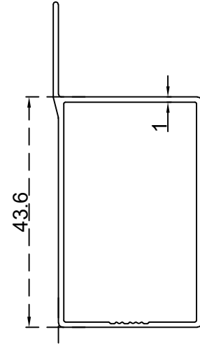
دفة (43.6 / 27.1) ملم مع كنت الرقم التسلسلي للصف: BLT3152 الوزن 0.423:(Kg/m)
