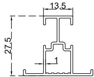
قاطع زجاج الرقم التسلسلي للصف: BLT145 الوزن 0.301:(Kg/m)
