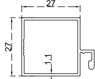
دفعه منخل (27 / 27) ملم الرقم التسلسلي للصنف: BLT361 الوزن 0.365:(Kg/m)
