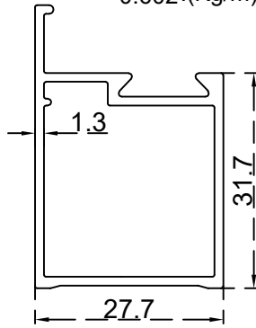
دفة زجاج (27.7 / 31.7) ملم الرقم التسلسلي للصف: BLT406 الوزن 0.489:(Kg/m)
