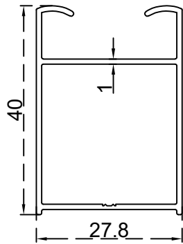
مجرى مكلمون سحب الرقم التسلسلي للصف: BLT3582 الوزن 0.388:(Kg/m)
