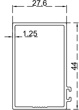
شوليف بي عادي ثقيل الرقم التسلسلي للصنف: BLT3148 الوزن 0.485:(Kg/m)
