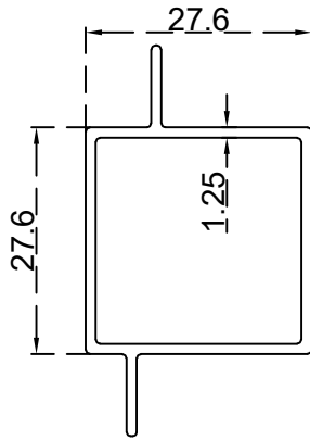
قاطع عرضي لتحتون 27.5 ملم الرقم التسلسلي للصنف: BLT3147 الوزن 0.426 : (Kg/m)
