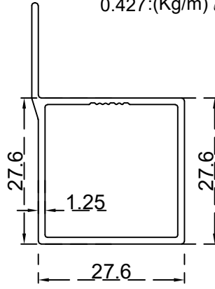
دفعه (27.6 / 27.6) ملم مع كنت الرقم التسلسلي للصنف: BLT3647 الوزن 0.422:(Kg/m)
