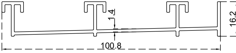
ارضية ثلاث مجاري الرقم التسلسلي للصنف: BLT844 الوزن 0.774:(Kg/m)
