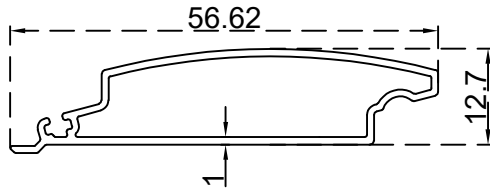
شلاف 50 ملم الرقم التسلسلي للصنف: ZD009B الوزن 0.328 : (Kg/m)
