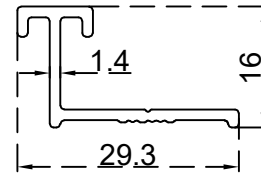
ارضية مجرى واحد الرقم التسلسلي للصنف: BLT3238 الوزن 0.210:(Kg/m)
