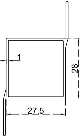
دفعه (27.6 / 27.6) ملم مع كنتين ثقيل الرقم التسلسلي للصنف: BLT373 الوزن 0.403:(Kg/m)
