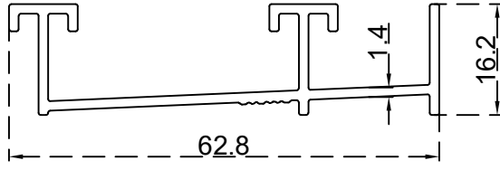
ارضية مجريين الرقم التسلسلي للصنف: BLT845 الوزن 0.501:(Kg/m)
