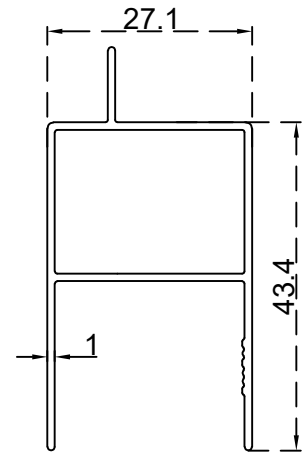
تحتون دقة 27.5 ملم الرقم التسلسلي للصنف: BLT843B الوزن 0.403 : (Kg/m)
