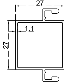
قاطع منخل الرقم التسلسلي للصنف: BLT362 الوزن 0.427:(Kg/m)
