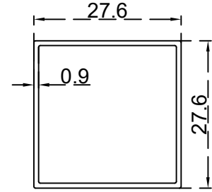
ساده (0.9*27.6*27.6) ملم الرقم التسلسلي للصنف: FG27.6X27.6X0.9 الوزن 0.261:(Kg/m)
