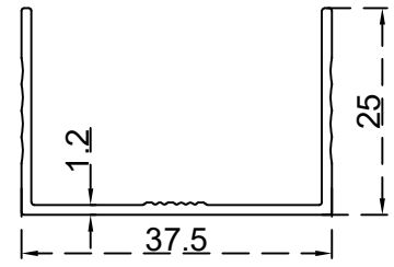
عليون مجرى واحد 25 ملم الرقم التسلسلي للصنف: BLT836 الوزن 0.272:(Kg/m)
